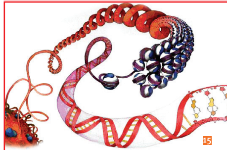
Le repliement de l'ADN dans le noyau, très compact, est réalisé par l'intermédiaire de structures organisées hiérarchiquement : nucléosome, fibre de chromatine, boucle, chromosome. La physique aide actuellement à mieux comprendre cette organisation, ses aspects mécaniques et les conditions de son fonctionnement.
